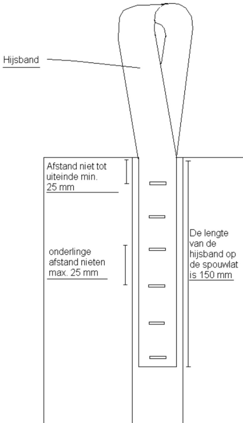
Figuur 2 (zijaanzicht)
